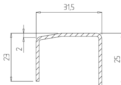
Усилитель Арт. № 207
