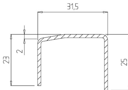
Усилитель Арт. № 207
