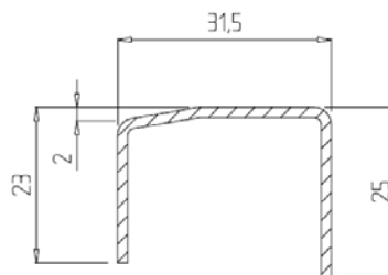
Усилитель Арт. № 207
